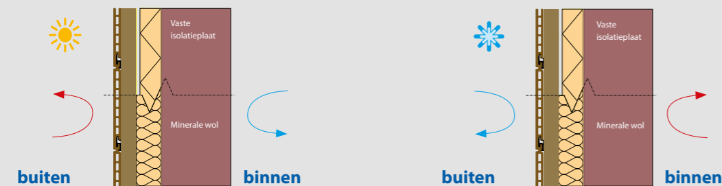
Geïsoleerde, geventileerde gevel die de zomerhitte buiten houdt, waardoor het binnen heerlijk koel blijft
